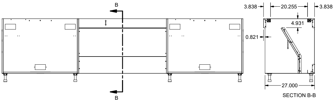
ADA Sink Space 48-60
