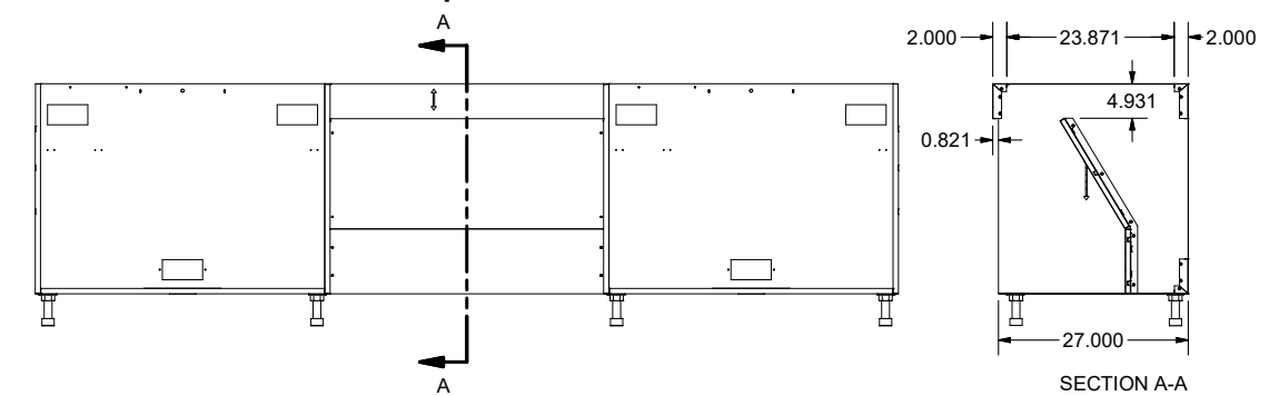
ADA Sink Space 36-39-42-45
